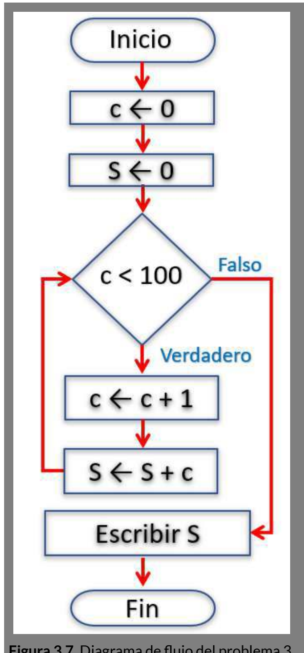
Figura 3.7. Diagrama de flujo del problema 3.
