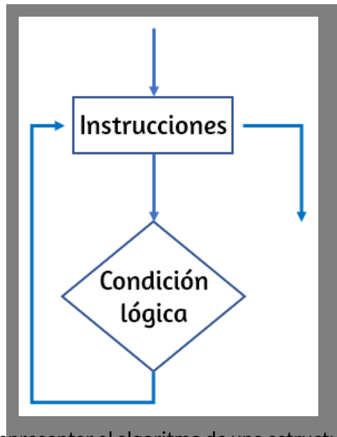
Figura 3.6. Forma de representar el algoritmo de una estructura iterativa Do-While.
