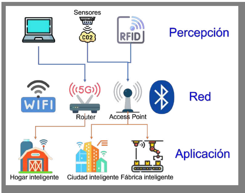
Figura 1.2. Arquitectura IoT, modelo de tres capas (imagen adaptada de Tasneem et al. [4]).
