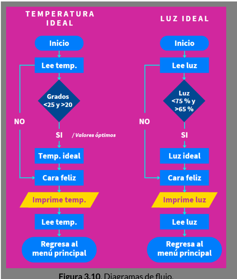
Figura 3.10. Diagramas de flujo.
